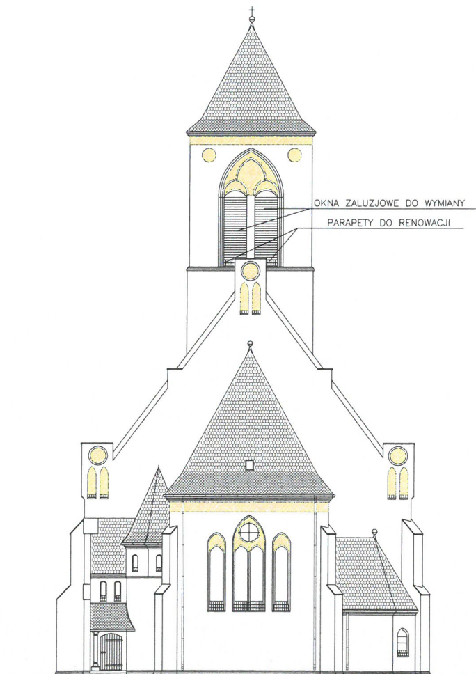
ELEWACJA POLNOCNIA
