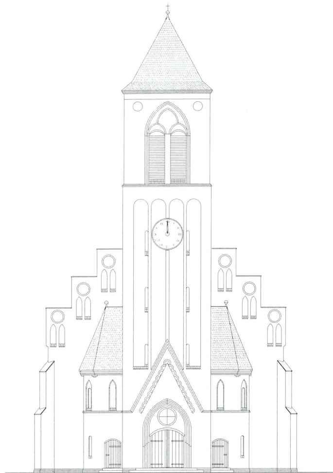
ELEWACJA POLUDNIOWA
