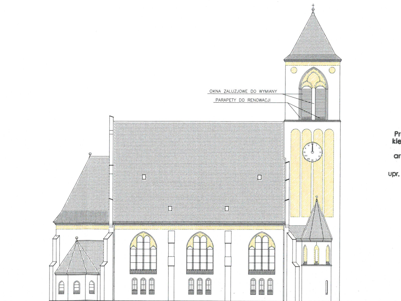
ELEWACJA ZACHODNIA
